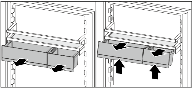
Fig. 79 ► 将 VarioBox 拉出至止挡。 ► 抬起 VarioBox 前部。 ► 向前取出 VarioBox。
