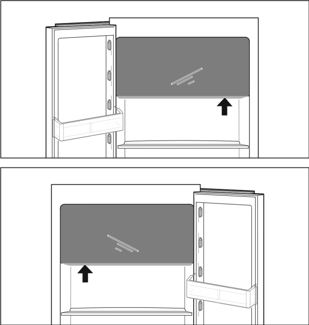
Fig. 75 打开冷冻室： ▶ 从底部进入把手区域。 ▶ 按下把手面板，同时向前拉开门。 关闭冷冻室： ▶ 关上门，同时从正面按下。 ▶ 门已卡紧。
