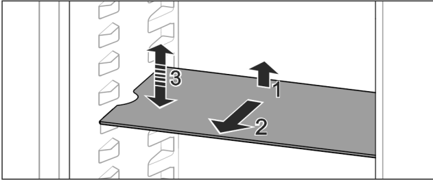
Fig. 80 ▶ 抬起搁板并向前拉出。 ▶ 使侧面凹口位于支撑位置。 ▶ 安装搁板：升降到任意高度并推入。 -或-
