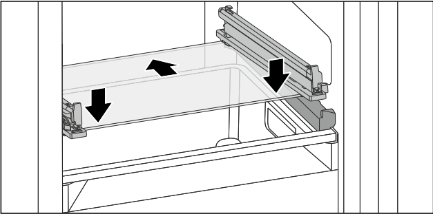
Fig. 71 可倾斜抽屉的玻璃隔板 ▶ 将玻璃隔板斜放在止动器后面。(参见 Fig. 71) ▶ 放低玻璃隔板。 ▶ 将玻璃板向后推入。 ▶ 玻璃隔板卡紧。
