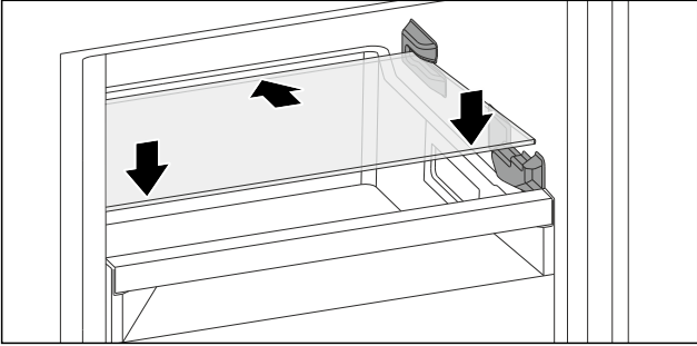
Fig. 73 玻璃隔板例图 ▶ 将玻璃隔板斜放在止动器后面。 ▶ 放低玻璃隔板。 ▶ 将玻璃板向后推入。
