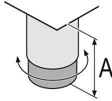
Fig. 76 Il piedino è regolabile da A = 115 mm (4 1/2 in) a 175 mm (6 7/8 in).*
