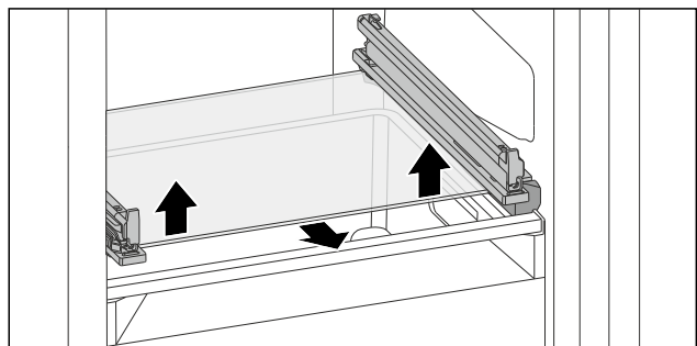
Fig. 133 可倾斜抽屉的玻璃隔板
