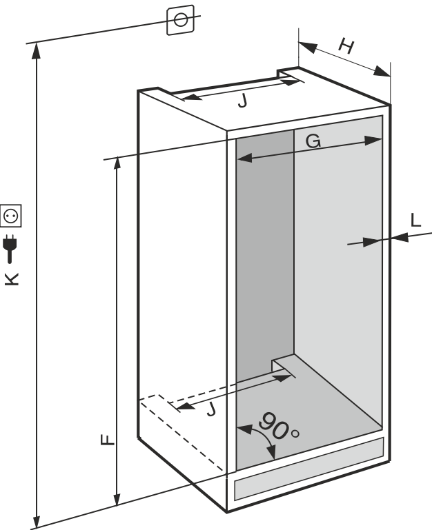
Fig. 3 (K): 最大2100 mm
