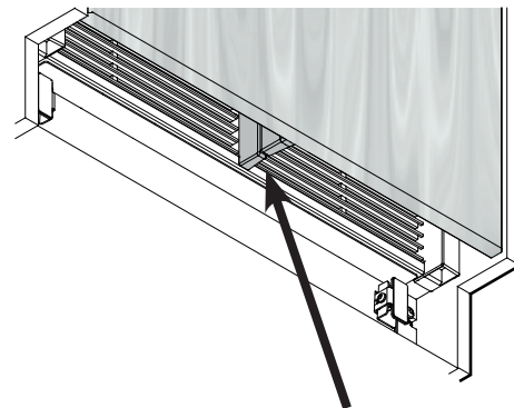
Spingere il filtro dell'acqua - con gli attacchi anteriori in posizione orizzontale - fino all'arresto, poi ruotarlo in senso orario, finché non si aggancia.
