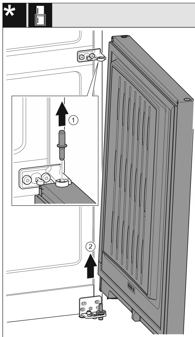
Fig. 11 Sans amortisseur de fermeture
