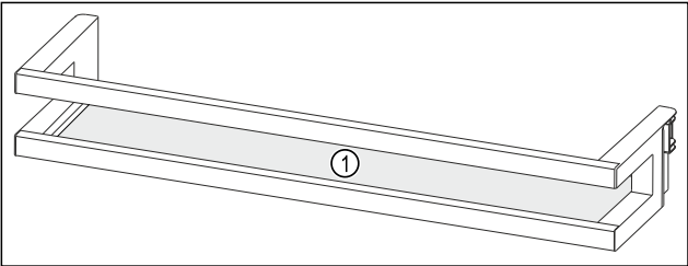
Fig. 100 门边存放架例图 (1) 搁板
