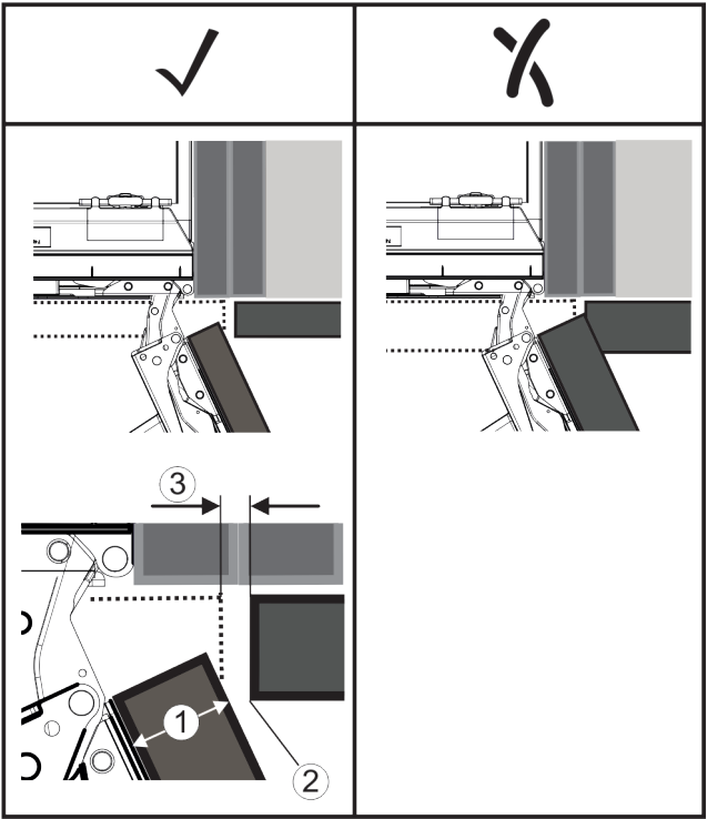
Fig. 20 (1) 正面厚度 (FD) (2) 边缘半径 (R) (3) 间隙尺寸 (S)
