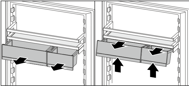
Fig. 103 ► 将 VarioBox 拉出至止挡。 ► 抬起 VarioBox 前部。 ► 向前取出 VarioBox。
