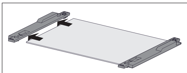
Fig. 129 带轨道和固定件的玻璃隔板
