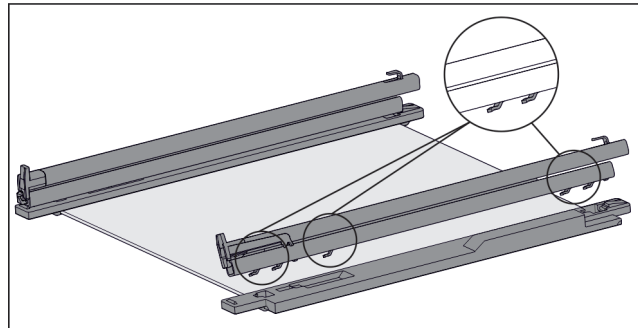
Fig. 108 Glasplatte mit Schienen und Halteteilen
