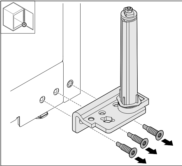
Fig. 40 ► Scharnierwinkel demontieren.
