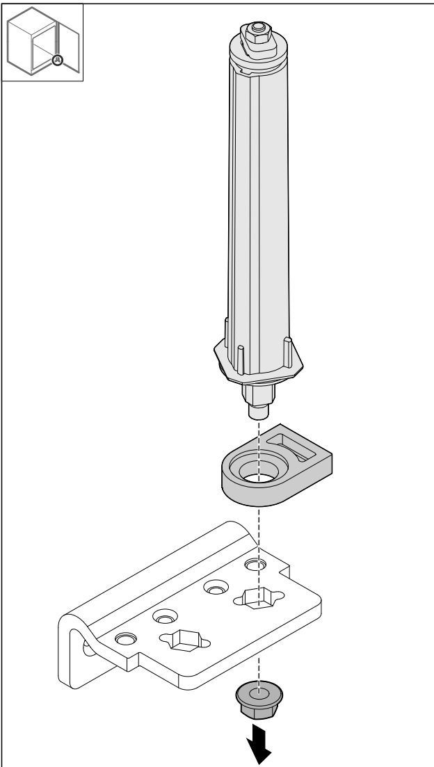
Fig. 40 ► Scharnierwinkel demontieren.
