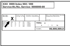
Fig. 3 Typenschild
