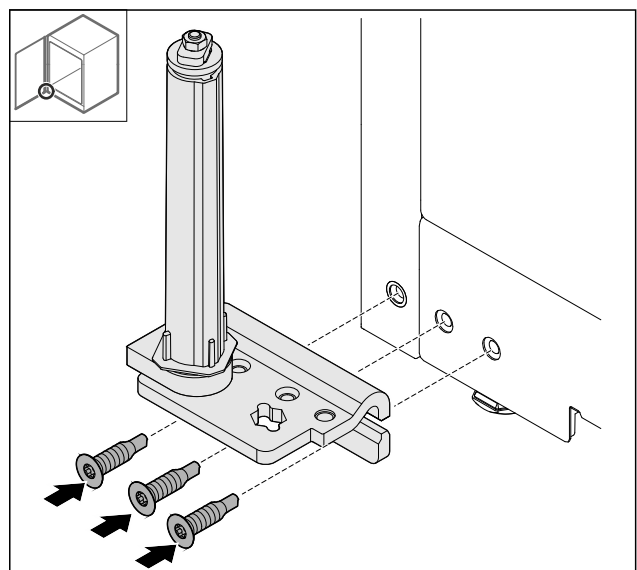
Fig. 42 Ansicht von unten: Fig. 42 (1) ► Schließsystem im Scharnierwinkel umsetzen und mit der Mutter fixieren.
