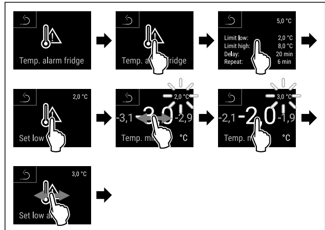
Fig. 152 Beispiel für die Einstellung der Temperaturuntergrenze, basierend auf einer eingestellten Gerätetemperatur von 5 °C.
