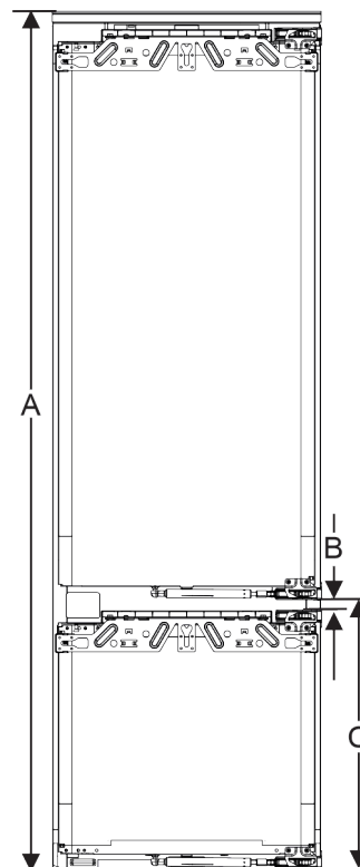
Fig. 70 Position des jointures sur une façade du meuble à deux portes
