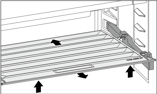
Fig. 145 ▶ 向后推抽屉盖。 ▶ 抬起抽屉盖前部。 ▶ 朝前方倾斜取出抽屉盖前部。
