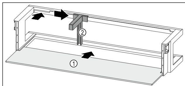
Fig. 96 带搁板的门边存放架
