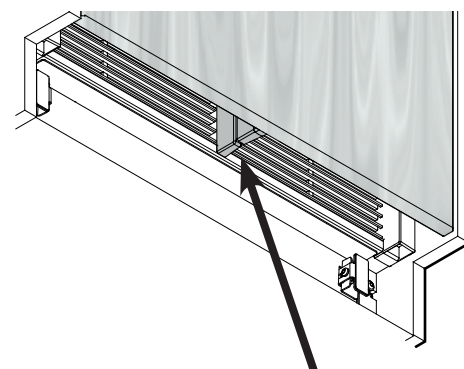
Insérer le filtre à eau – avec les picots avant en position horizontale – jusqu'à la butée et tourner dans le sens horaire jusqu'à ce qu'il s'enclipsse.
