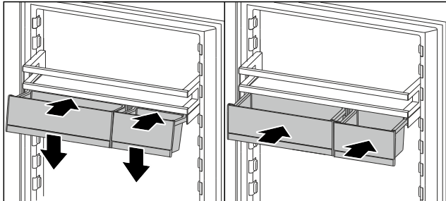
Fig. 82 ► 将 VarioBox 倾斜放在门边存放架的滑条上。 ► 放低 VarioBox。 ► 推入 VarioBox。
