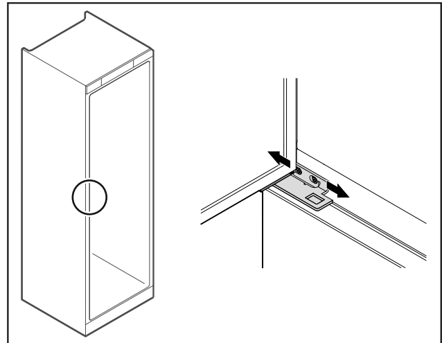
Fig. 60 Kühlteil
