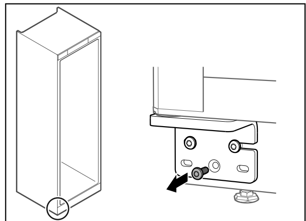
Fig. 61 Gefrierteil
