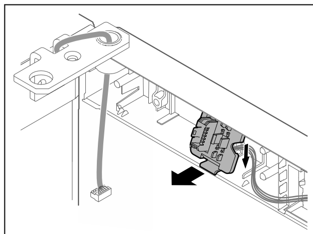
Fig. 11 Монтажную позицию держателя штекера можно повернуть на 180°.*
