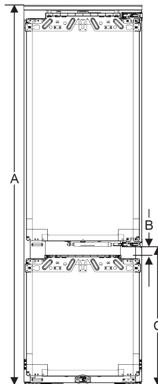
Fig. 63 Fugenlage Kellerfach
