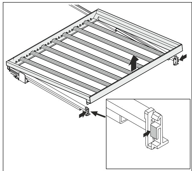
Fig. 98 Przykładowa prezentacja
