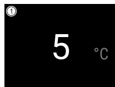
Fig. 16 Wskaźnik statusu*
