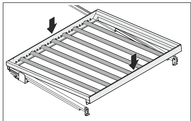
Fig. 99 Przykładowa prezentacja
