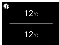
Fig. 17 Wskaźnik statusu*
