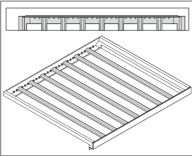
Fig. 94 Rozmieszczenie listew dla maksymalnej liczby butelek.
