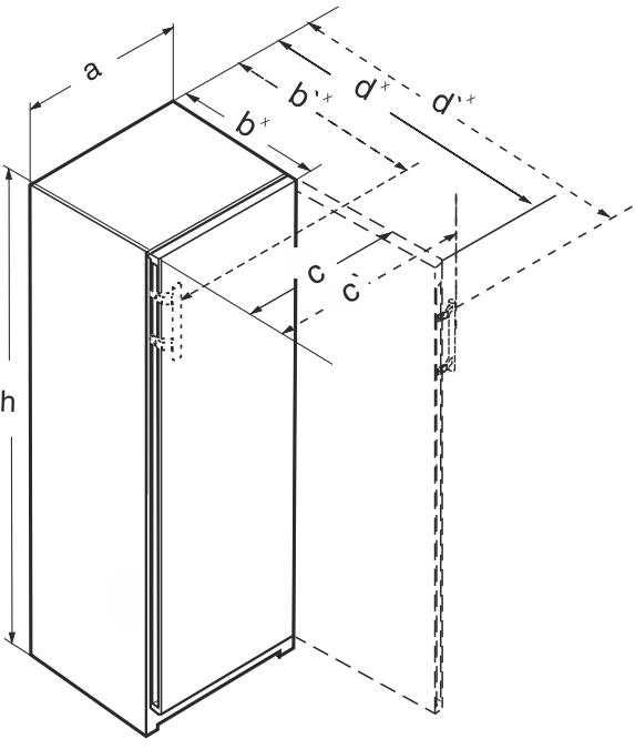
Fig. 2 (a) 冰箱宽度 (b) 冰箱深度 (c) 打开门时的冰箱宽度 (d) 打开门时的冰箱深度 (f) 带扶手的尺寸
