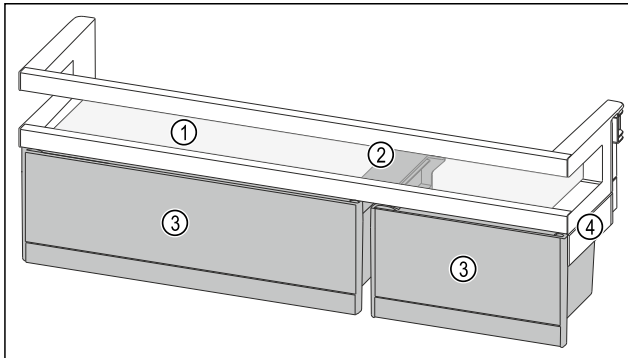
Fig. 105 Beispielhafte Darstellung Türabsteller mit VarioBoxen* (1) Abstellfläche (3) VarioBoxen (2) Halteteil für Vario-Boxen (4) Seitenteil
