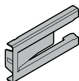
Cache
