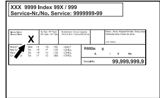
Fig. 6 Typenschild
