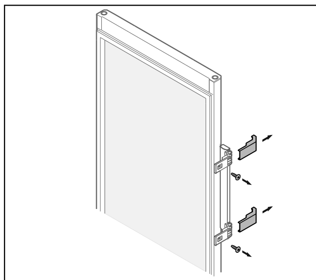
Fig. 20 Glastür*
