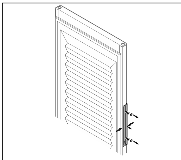
Fig. 19 Geschäumte Tür*
