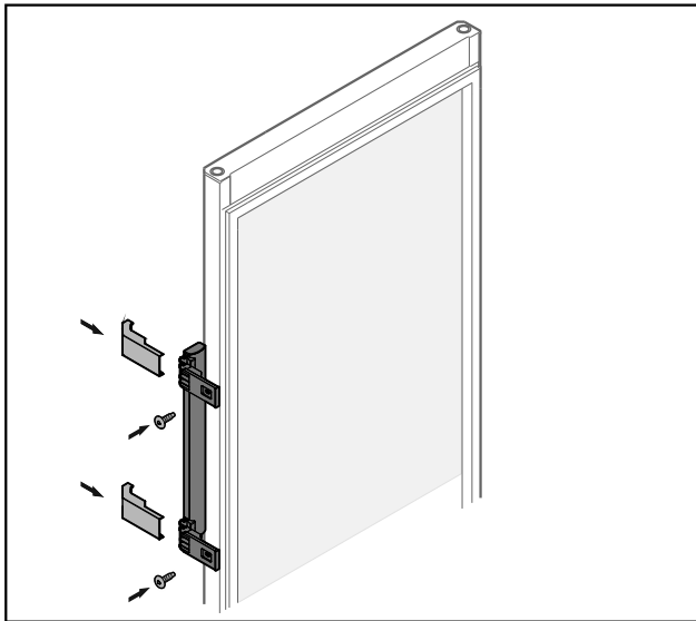
Fig. 23 Glastür*
