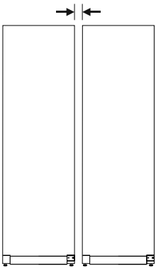
Fig. 49 Installazione Side-by-Side
