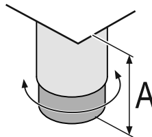
Fig. 41 Der Stellfuß ist von A = 115 \text{ mm} (4 1/2 in) bis 175 \text{ mm} (6 7/8 in) verstellbar.
