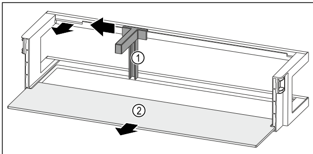
Fig. 133 Türabsteller mit Flaschenhalter und Abstellfläche
