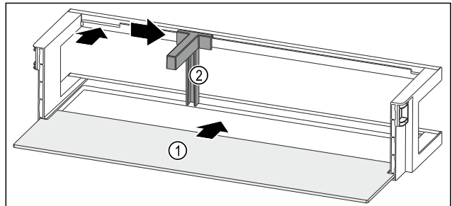
Fig. 136 Türabsteller mit Abstellfläche
