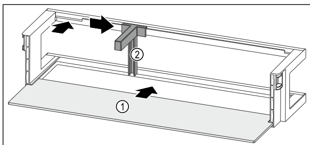
Fig. 121 Balconcino controporta con ripiano
