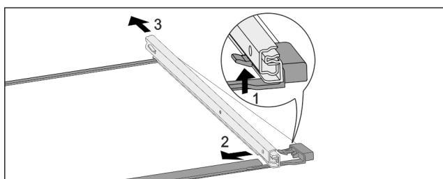
Fig. 179 Ripiano in vetro con guide
