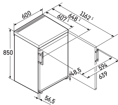
Rci 1621 Rsdci 1621 Rsdci 1620 Rdi 1621 Rci 1620 Rdi 1620 [mm]
