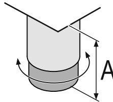
Fig. 10 Опорная ножка регулируется от A = 115 мм (4 1/2 in) до 175 мм (6 7/8 in).
