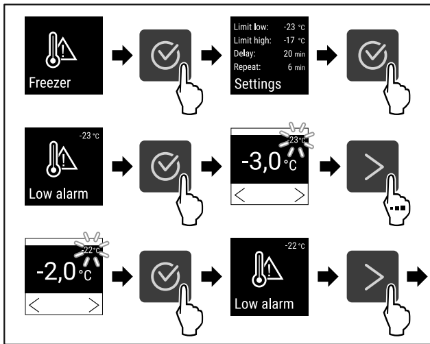
Fig. 46 Beispiel für die Einstellung der Temperaturuntergrenze, basierend auf einer eingestellten Gerätetemperatur von -20 °C.
