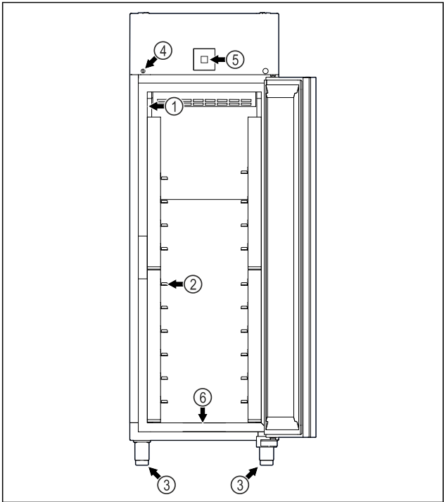
Fig. 1 Representación a modo de ejemplo (1) Placa de características (2) Riel para bandejas (3) Pata de ajuste (4) Cierre (5) Controles e indicación de temperatura (6) Orificio de vaciado para el agua de limpieza
