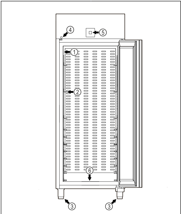
Fig. 2 Representación a modo de ejemplo (1) Placa de características (2) Riel para bandejas (3) Pata de ajuste (4) Cierre (5) Controles e indicación de temperatura (6) Orificio de vaciado para el agua de limpieza
