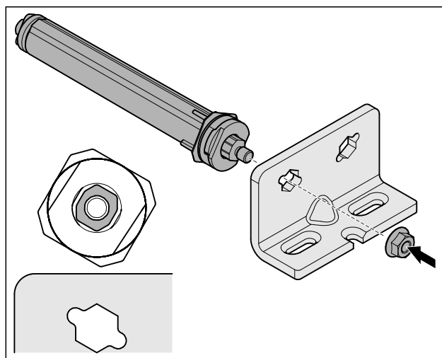
Fig. 16 Montaje de las bisagras a la izquierda
