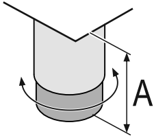
Fig. 52 Il piedino è regolabile da A = 150 mm (6 5/16 in) a 180 mm (7 1/16 in).*
