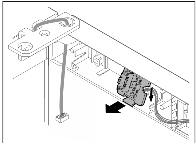
Fig. 15 La posizione di montaggio del supporto della spina può essere ruotata di 180°.*
