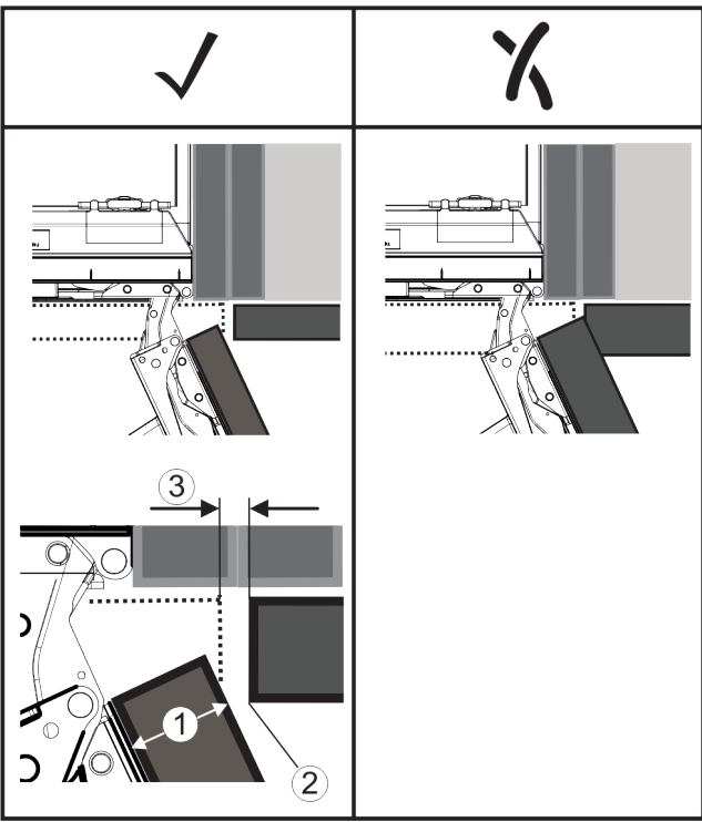
Fig. 67 (1) 正面厚度 (FD) (2) 边缘半径 (R) (3) 间隙尺寸 (S)
