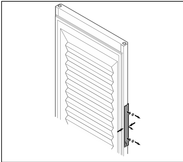
Fig. 9 Geschäumte Tür
