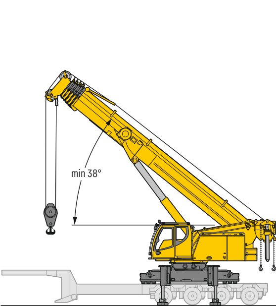
Boom lift to min. 38° on low loader Relevage à 38° minimum sur la remorque surbaissée
