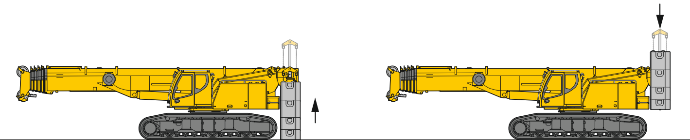
Assembly superstructure ballast Montage du contrepoids de la partie tournante
