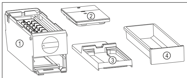
Fig. 107 Componenti dell'EasyTwist-Ice
