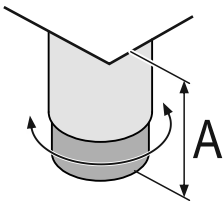
Fig. 76 Der Stellfuß ist von A = 115 \text{ mm} (4 1/2 in) bis 175 \text{ mm} (6 7/8 in) verstellbar.*
