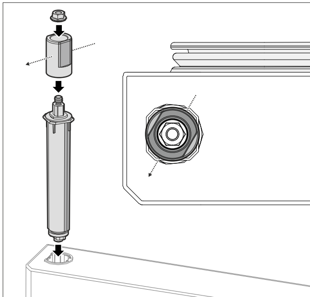
Fig. 56 Linksanschlag
