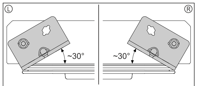
Fig. 61 Tür von unten
