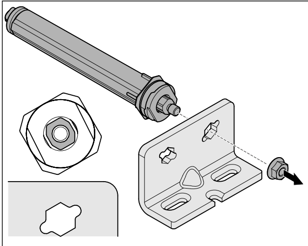
Fig. 24 Rechtsanschlag
