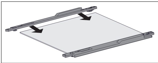
Fig. 120 Glasplatte mit Halteteilen
