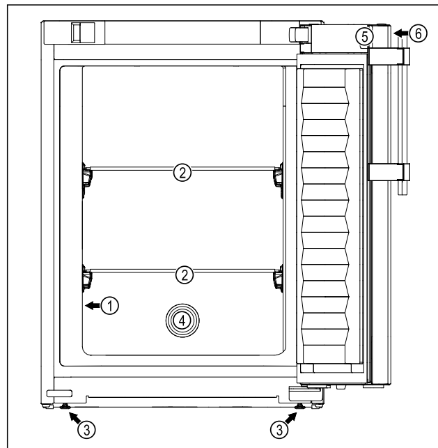
Fig. 1 Примерное изображение: Устройство со стеклянными пластинами и устройством со стеклянными пластинами и выдвижным ящиком
