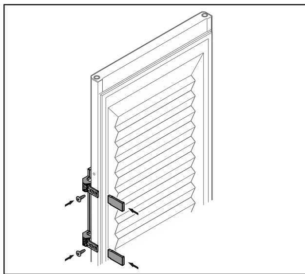
Fig. 23 Запененная дверь*
