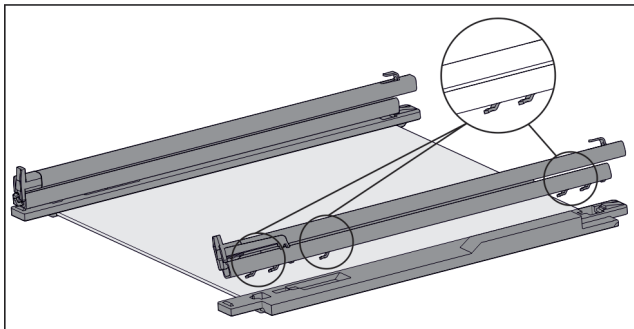
Fig. 118 Skleněná deska s kolejničkami a přídržnými díly
