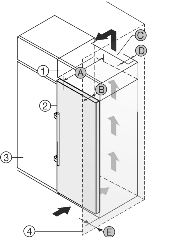
Fig. 5 (1) 附加柜 (2) 冰箱 (3) 餐柜 (4) 墙壁 (A) 冰箱深度 (B) 门深度 (C) 通风横截面 (D) 冰箱背面间距 (E) 到冰箱侧面的间距
