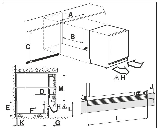
Fig. 3 Beispielhafte Darstellung: ..pr (A) Nischenbreite (C) Nischenhöhe (B) Nischentiefe (H) Lüftungsquerschnitt
