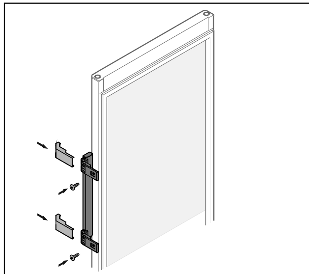
Fig. 25 Glass door*
