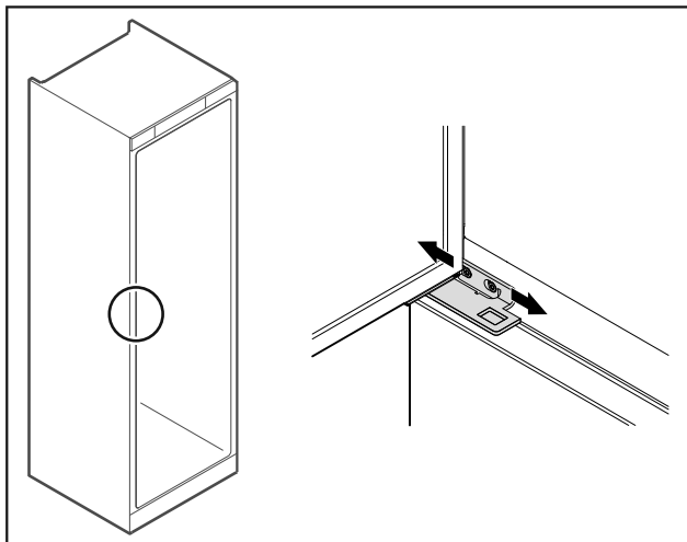
Fig. 61 Kühlteil
