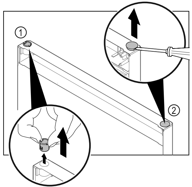
Fig. 30 Gefrierteiltür
