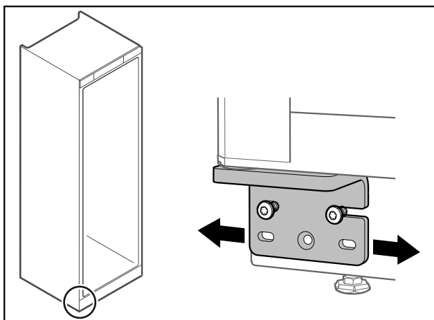
Fig. 63 Gefrierteil
