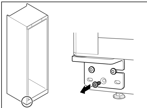
Fig. 62 Gefrierteil
