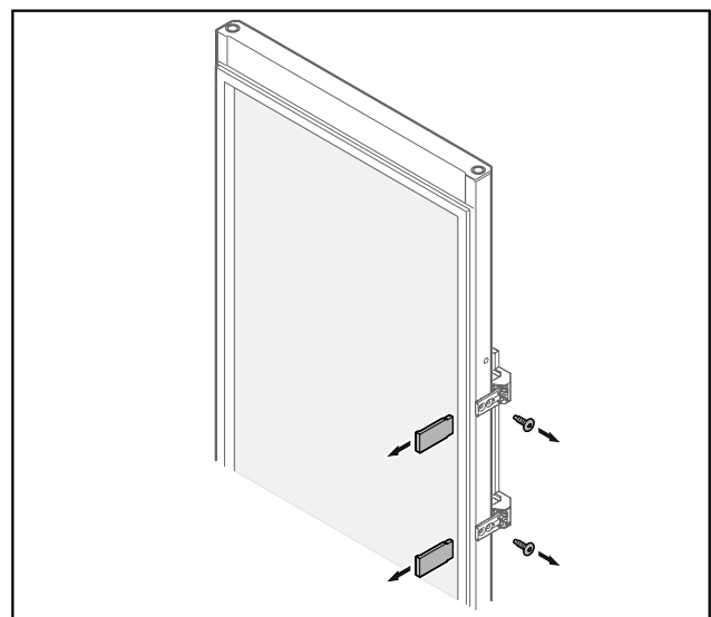
Fig. 26 Glastür*
