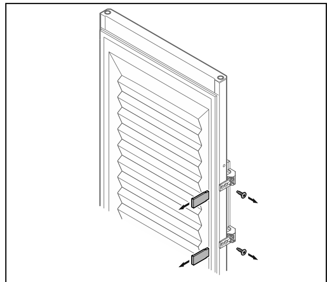
Fig. 25 Geschäumte Tür*
