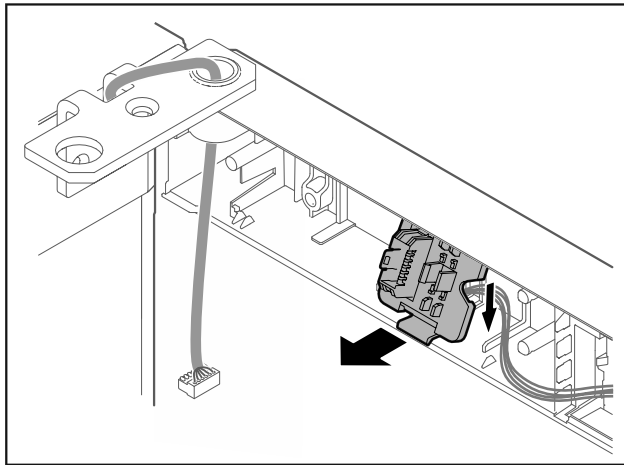
Fig. 15 Монтажную позицию держателя штекера можно повернуть на 180°.*
