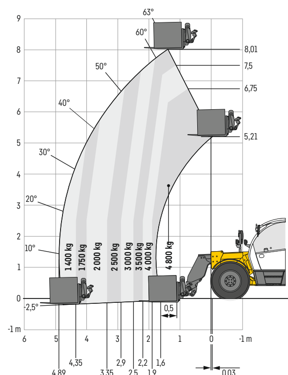
T 48-8s avec blocage de l'essieu pendulaire
