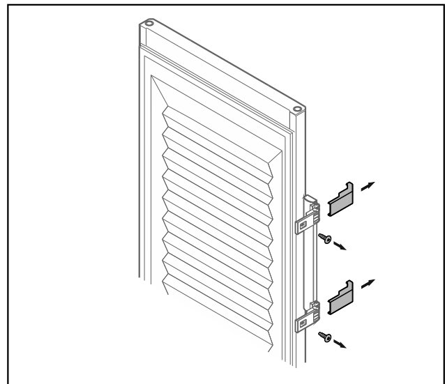
Fig. 25 Porta in materiale espanso*
