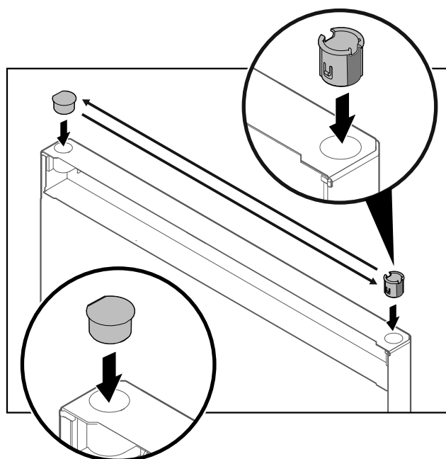
Fig. 31 Porta del vano congelatore
