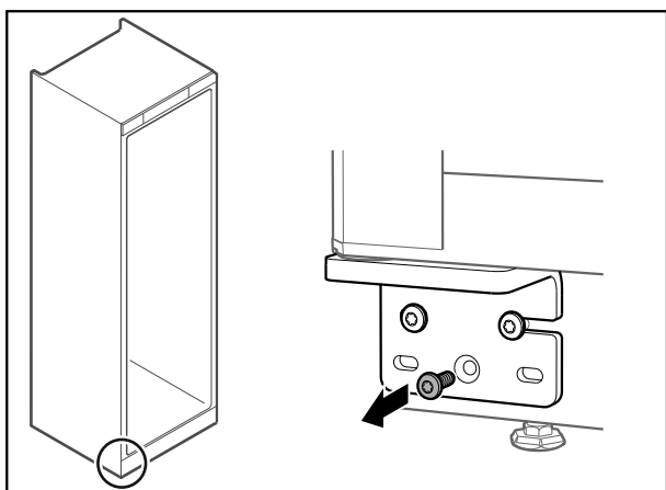
Fig. 62 Vano congelatore
