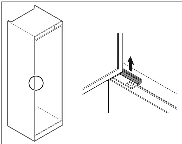
Fig. 60 Vano frigorifero
