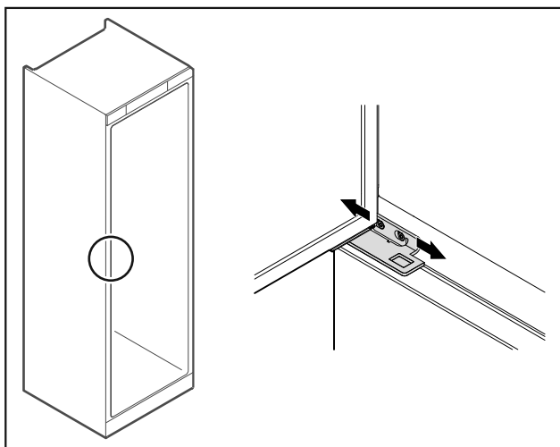
Fig. 61 Vano frigorifero
