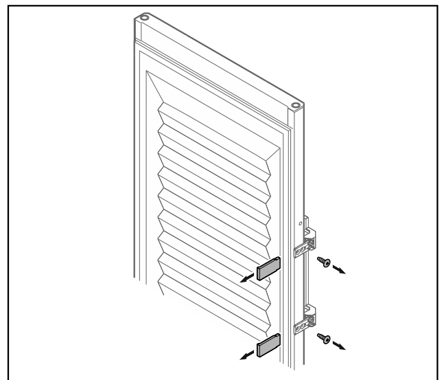
Fig. 20 Geschäumte Tür
