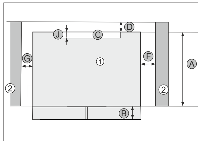
Fig. 9 Draufsicht
