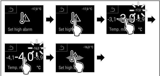
Fig. 143 Exemple pour le réglage du seuil inférieur de température en se basant sur une température d'appareil définie de -20 °C.
