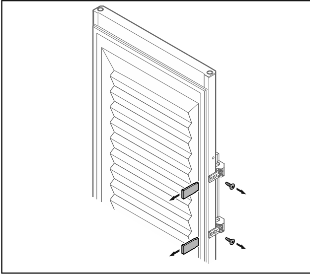
Fig. 19 Intérieur de porte moussé
